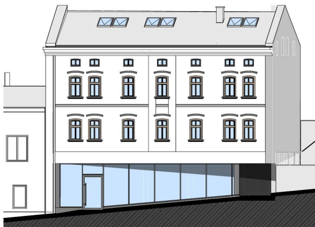
Elewacja frontowa - od ulicy Bytomskiej
